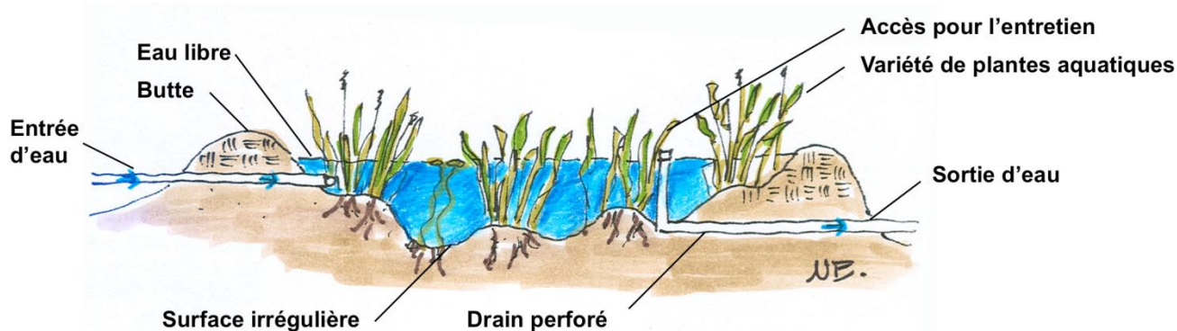
Figure 12. Marais filtrant à écoulement des eaux sur la surface. Illustration : N. Bédard
